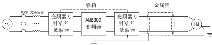
图 3-9 射频干扰措施
